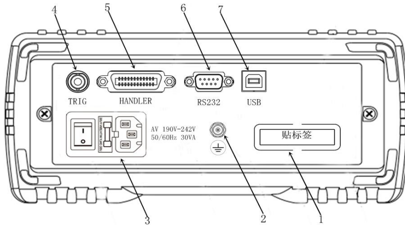
图2-4后面板
